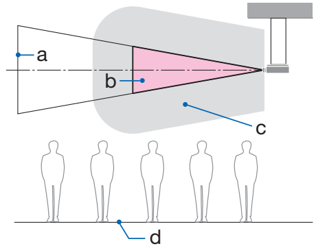
a : スクリーン / b : 侵入禁止領域 / c : 保安領域 / d : 床面
