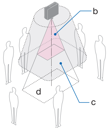
b : 侵入禁止領域 / c : 保安領域 / d : 床面
