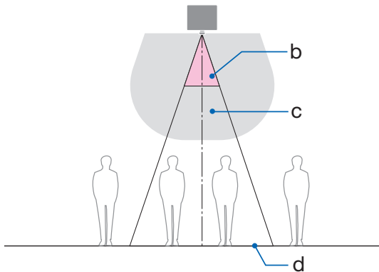
b : 侵入禁止領域 / c : 保安領域 / d : 床面
