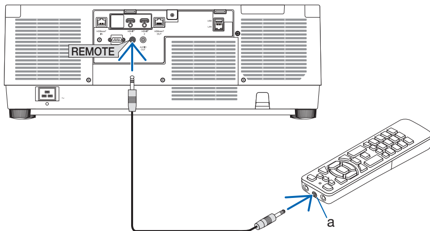
a: リモコンケーブル接続端子
