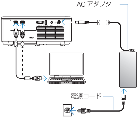
【接続図】
